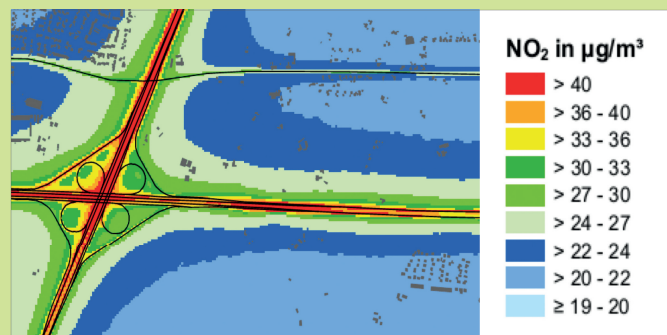
Beispieldarstellung einer Immissionsprognose für NO 2
